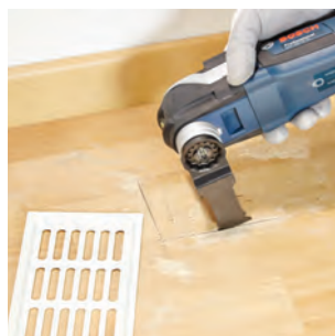
穿刺切割層壓板， 例如：安裝通風格柵
